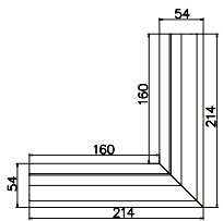
BV7600Y Ecke 90° (Intern) Eloxiertes Aluminium. Code: C7602Y
