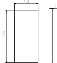
ENDE-DECKEL Eloxiertes Aluminium Code: BV7601K
