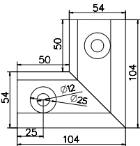
BV7600 Ecke 90° (Extern) Eloxiertes Aluminium. Code: C7601
