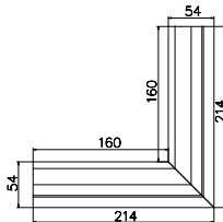
BV7600Y Ecke 90° (Extern) Eloxiertes Aluminium. Code: C7601Y
