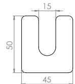
SHIMS Edelstahl Code: SH7600 (Dicke auf Anfrage)
