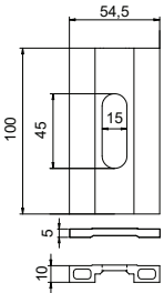
ENTWÄSSERUNG- SPLATTE Eloxiertes Aluminium Code: BV7600DP/5, BV7600DP/10
