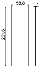
ENDE-DECKEL Eloxiertes Aluminium Code: BV7601YK
