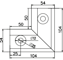
BV7600 Ecke 90° (Intern) Eloxiertes Aluminium. Code: C7602
